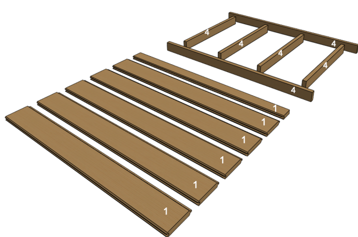
ETAPE A- Solivage et plancher
