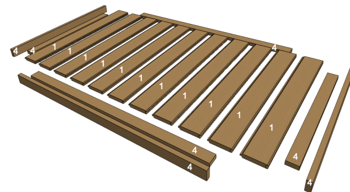
ETAPE C- TOIT
