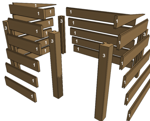
ETAPE B- Murs
